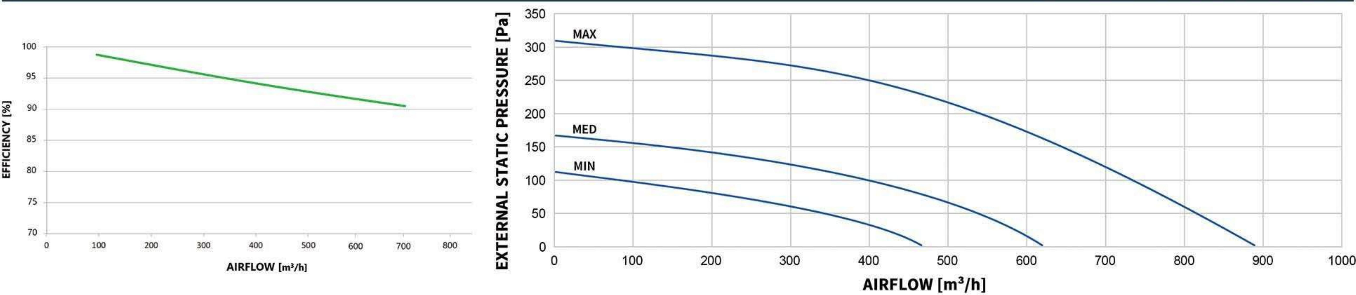
MODEL: W700-ERV-B-Z-EC
